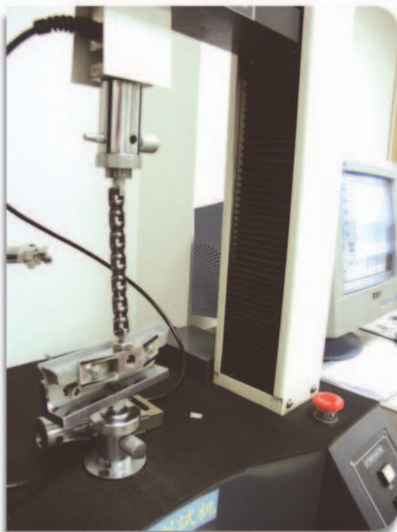
Tensile Strength 拉力測試
